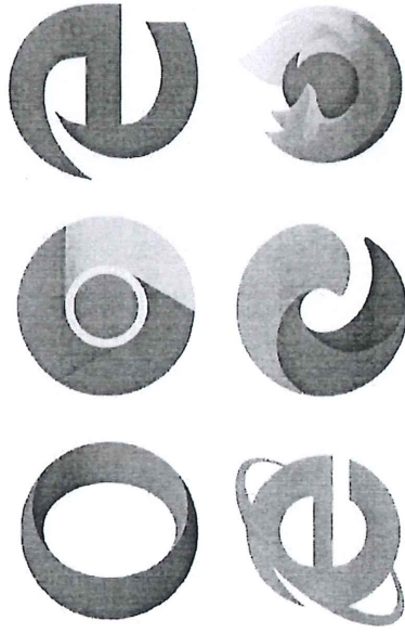
Web browser
